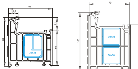
Рама 80 мм арт. №101.214 усилитель арт. №113.271 усилитель арт. №113.302
