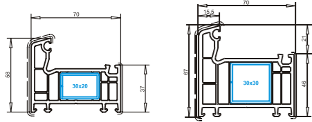
Рама 58 мм арт. №101.207 усилитель арт. №113.019
