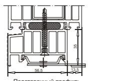
Подставочный профиль арт. №110.011 Анкер, арт. №141.138
