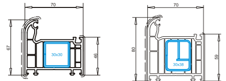
Рама 67 мм арт. №101.233 усилитель арт. №113.025
