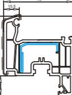
Створка 80 мм арт. №103.232 усилитель арт. №113.292 усилитель цветной створки арт. №113.294 усилитель сдвижной двери арт. №113.295
