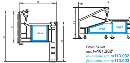
Рама 95 мм арт. №101.218 усилитель арт. №113.025
